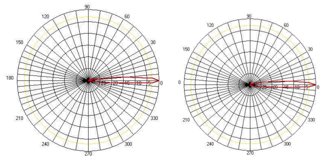
E-plane
