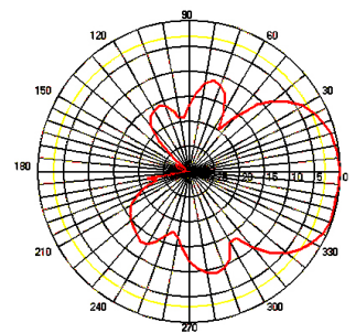
H-Plan@1800MHz
