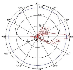
870~960MHz: VPol
