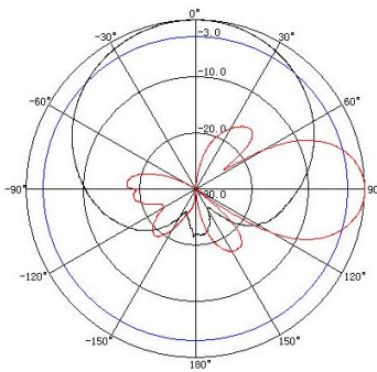
824-896MHz: VPol
