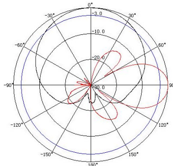
870-960MHz: VPol
