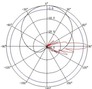
824~896MHz: VPol
