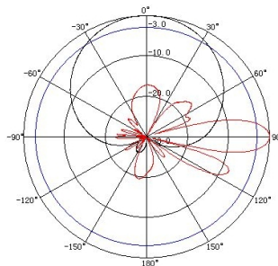
870~960MHz: VPol
