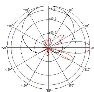
824~896MHz: VPol
