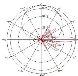
1710~1880MHz: ±45° Pol.
