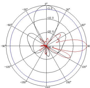
824~896MHz: VPol
