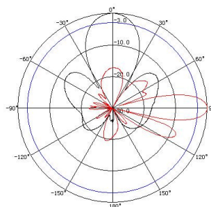
870~960MHz: VPol
