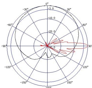
806~896MHz: VPol
