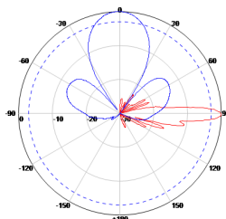
1850~1990MHz: ±45° Pol.
