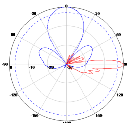
1710~1880MHz: ±45° Pol.
