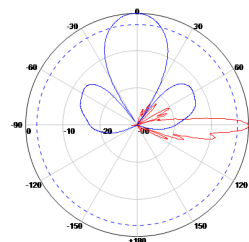
1920~2170MHz: ±45° Pol.
