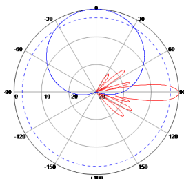
806~896MHz: ±45° Polarization
